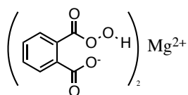
mono peroxyphthalate (MMPP)
