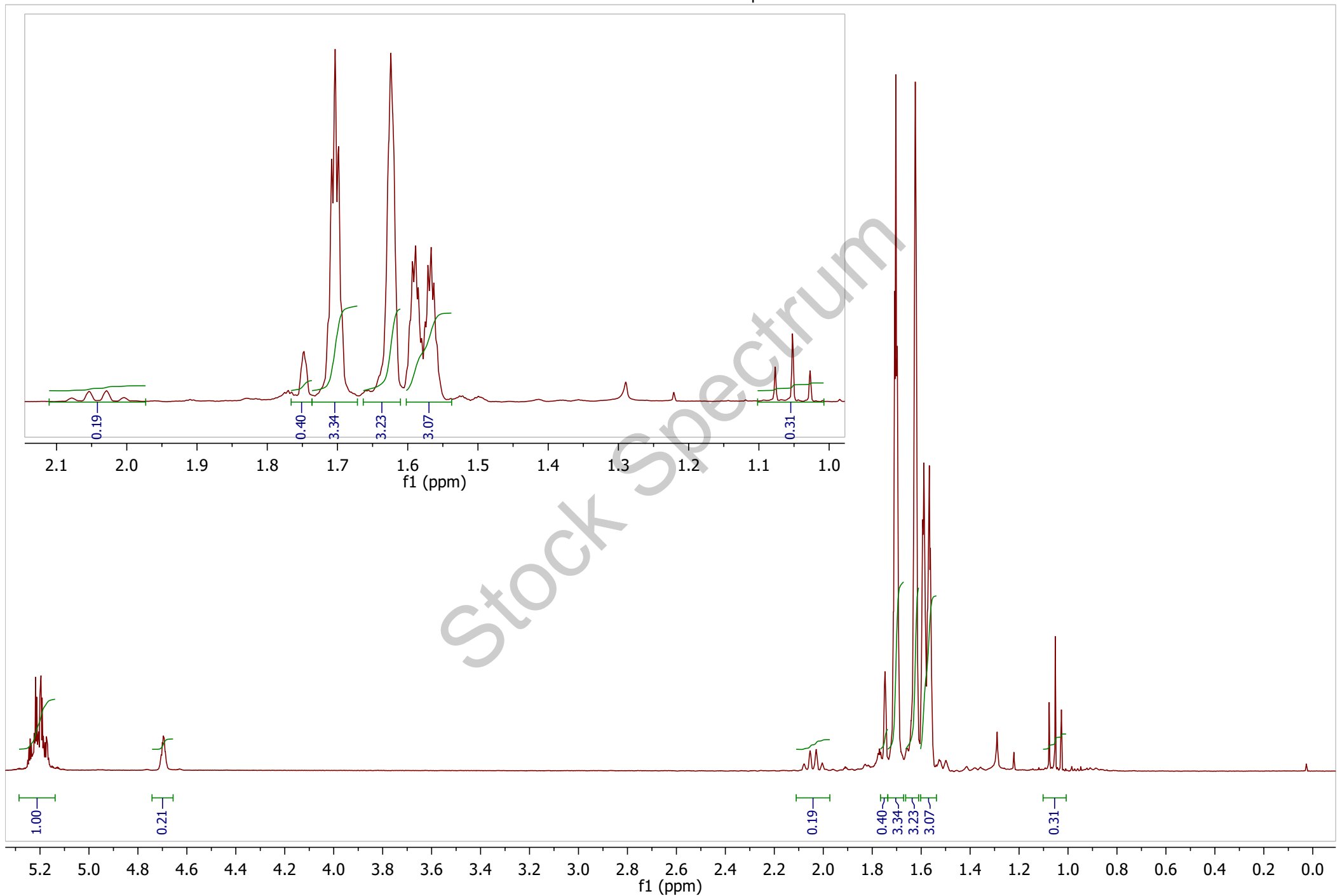
CHEM 344 E1 Stock 1H-NMR Spectrum
