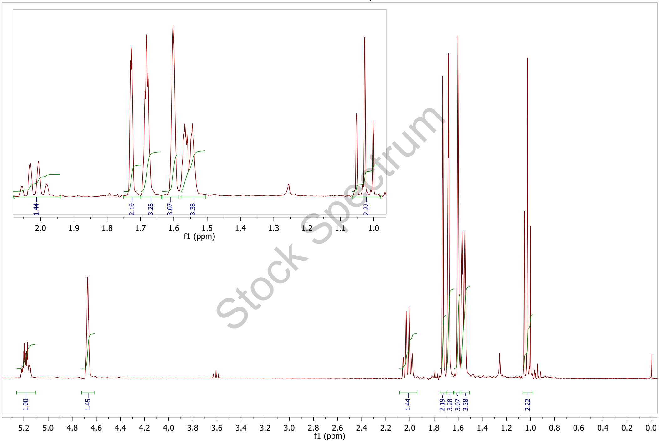
CHEM 344 E2 Stock 1H-NMR Spectrum
